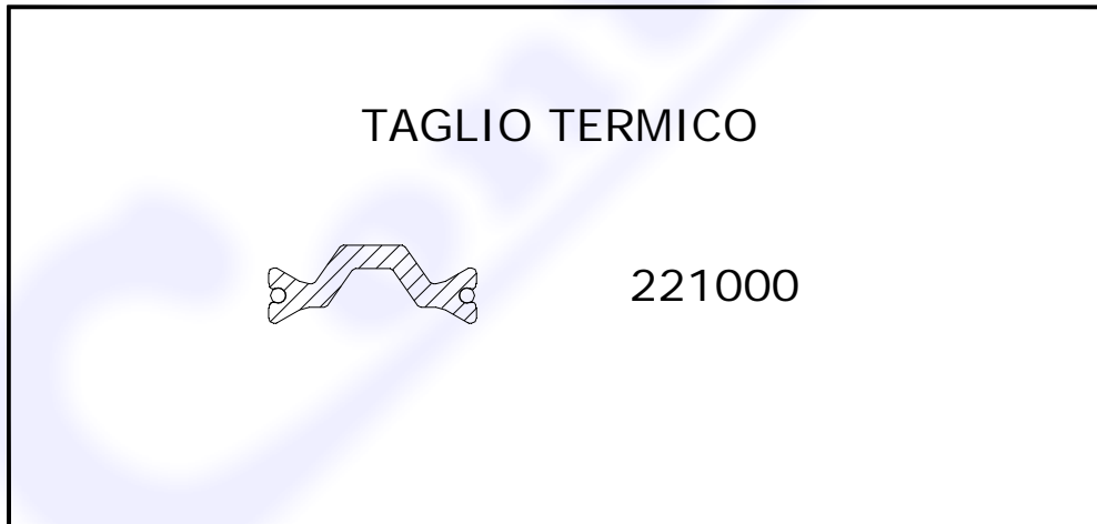
Fig. 4b: Dettagli del taglio termico del campione pervenuto e sottoposto a prova (dimensioni nominali dichiarate, espresse in mm)
