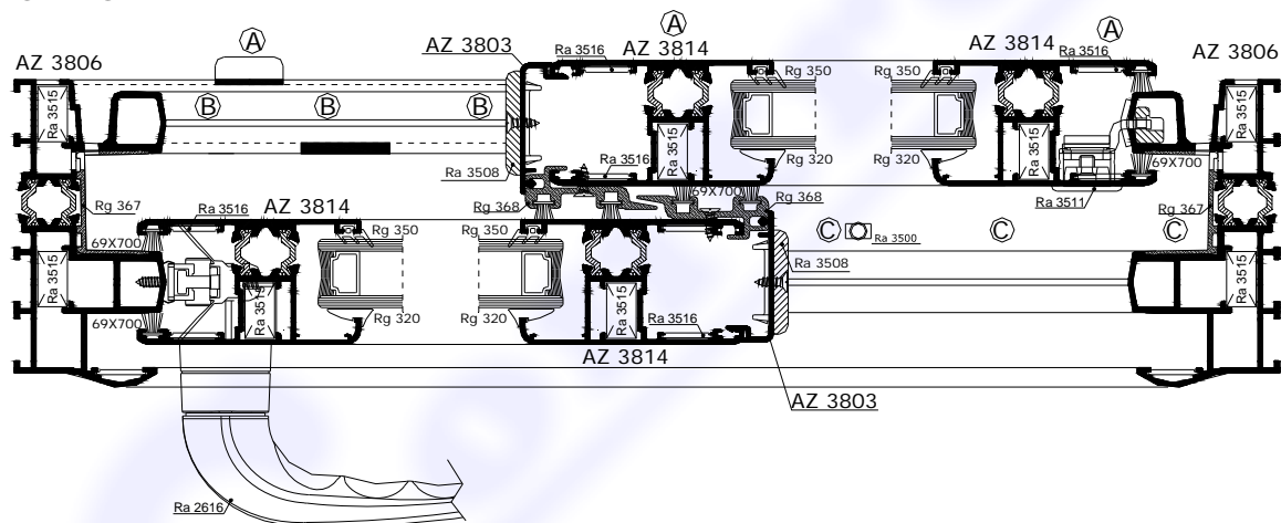
Fig. 2b: sezione orizzontale del campione pervenuto e sottoposto a prova (dimensioni nominali dichiarate, espresse in mm)
