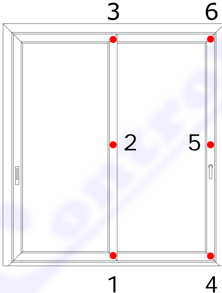
Fig. 5: Assetto sperimentale prova di resistenza al carico del vento: schema di posizionamento dei trasduttori (vista interna)
